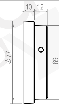
TAPPO (plug)
