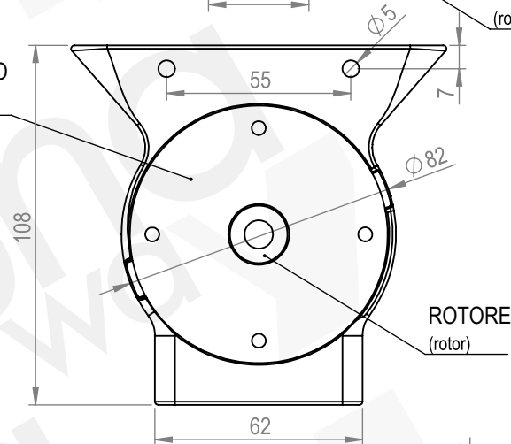
ROTORE (rotor)
