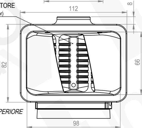
TAPPO (plug)
