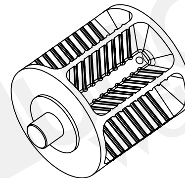
ROTORE (rotor)
