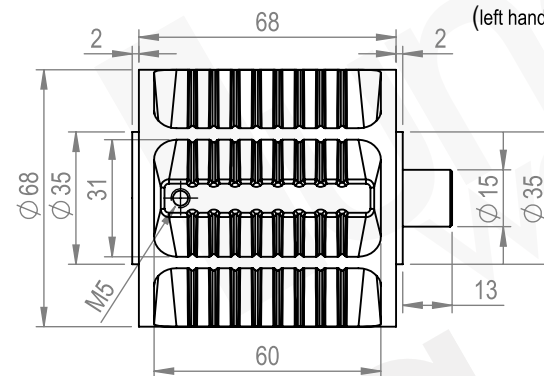
ROTORE (rotor)
