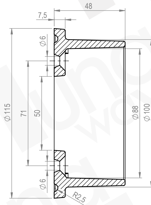
SECTION A-A SCALE 2 : 3
