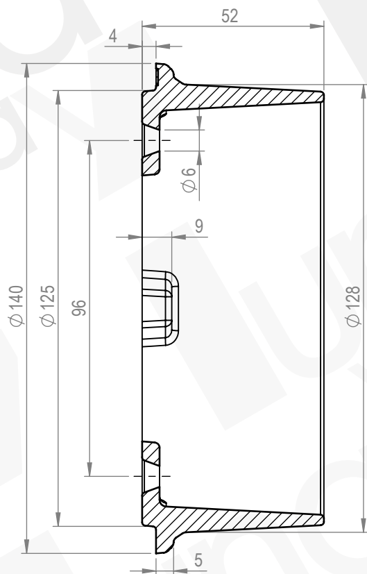
SECTION A-A SCALE 2 : 3
