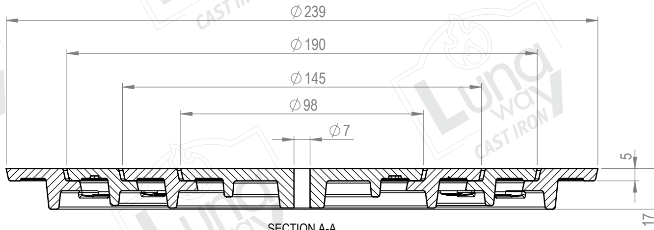
SECTION A-A SCALE 2 : 3
